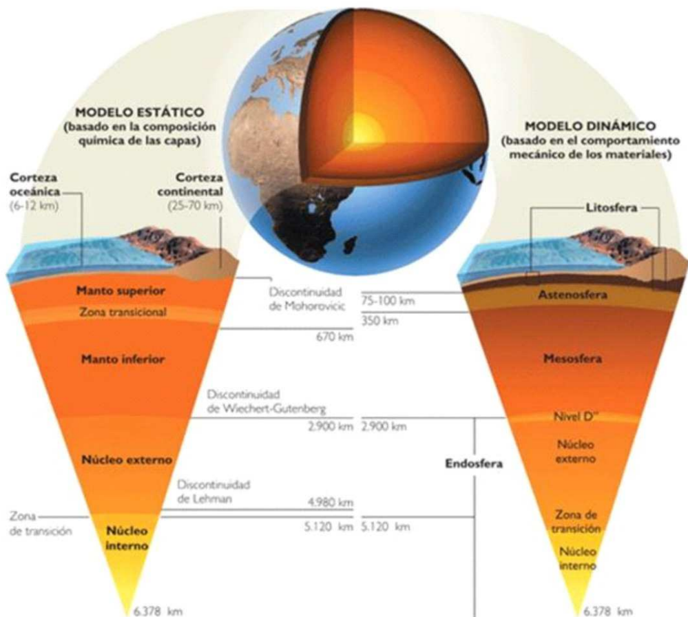
Figura 1: Esquema mostrando las distintas capas de la Tierra, en cuanto a su composición (imagen izquierda) y las capas mecánicas(imagen derecha). (Tomada de http://ciencias.us/ )
