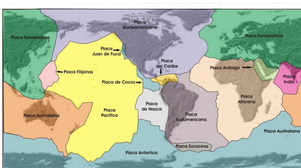
Figura 2: División de la superficie de la Tierra en placas.
