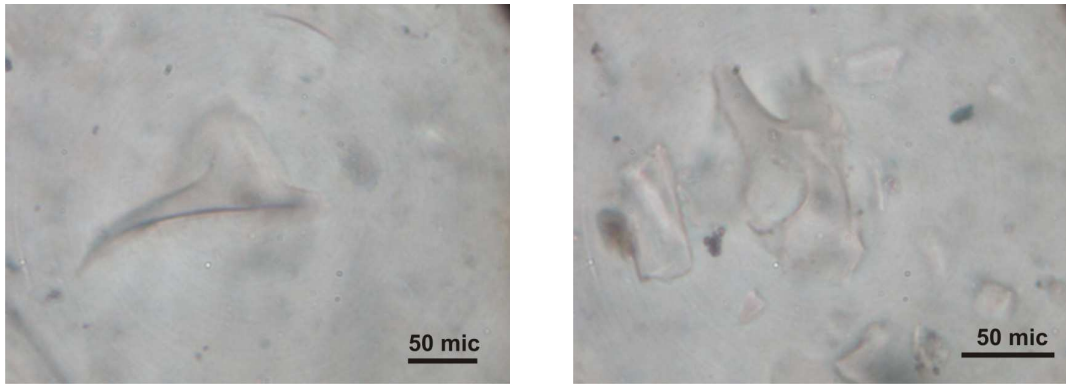
Figura 2: Fotografías de cenizas volcánicas que cayeron en Buenos Aires en junio 2011 (volcán Puyehue-Cordón Caulle), vista al microscopio de polarización. Puede observarse las formas puntiagudas que presentan y las formas redondeadas que marcan claramente que han sido las paredes de las burbujas, tal como se explicaba en el texto y la figura 1. (Microfotografía de la Dra. S. Alonso)
