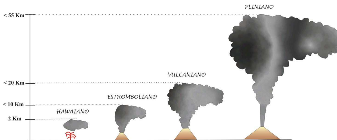
Figura 6: Cuadro de los distintos estilos eruptivos y la altura que puede alcanzar la columna eruptiva.
