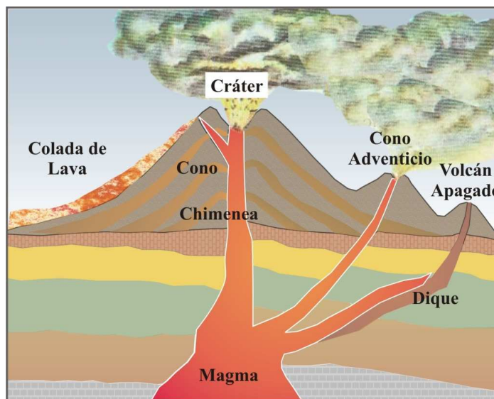
Figura 5: esquema de un volcán.
