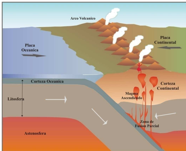
Figura 4: Conforme una placa oceánica desciende hacia el manto, el agua y otros compuestos volátiles desaparecen de las rocas de la corteza subductada. Estos volátiles disminuyen la temperatura de la fusión de las rocas del manto lo bastante como para generar fusión
