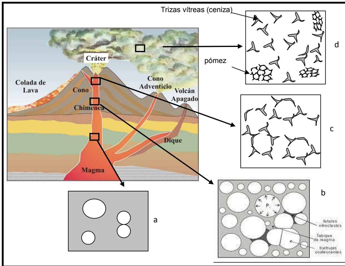
Figura 1: Representación del origen de las cenizas en los volcanes (a) porción del magma (en gris) con formación de burbujas (en blanco) producidas por pérdida de presión; (b) aumento de exsolución de burbujas (círculos blancos) del magma (en gris) mostrando los tabiques (remarcado en negro) que se forman al crecer las burbujas y disminuir el espacio entre ellas (futuras trizas vítreas que en conjunto son denominadas como ceniza volcánica al ser eyectadas por el cráter); (c) fragmentación de los tabiques (en gris) que existe entre burbujas dando lugar a partículas puntiagudas denominadas trizas vítreas o ceniza; (d) porción de la nube donde se observan las trizas eyectadas (que darán lugar a nubes de cenizas) junto a porciones que no se fragmentaron (pómez).
