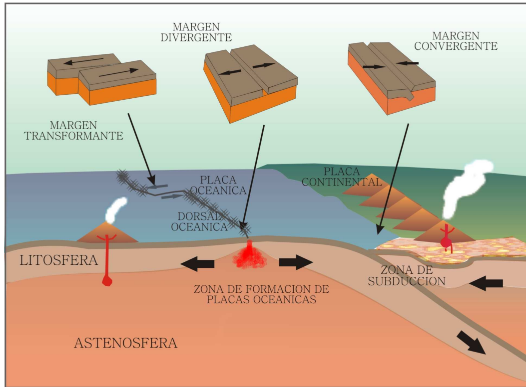
Figura 3: Tipos de bordes entre placas tectónicas.
